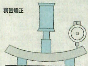
【作業能力】 □:10~100mm 長さ6m ○:8~100mm 長さ6m 【矯正精度】0.05~0.3mm
